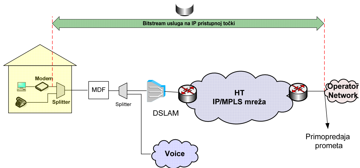
Slika 16. Veleprodajni širokopojsni pristup za pružanje VoIP usluge na IP razini u slučaju kada krajnji korisnik ostvaruje Osnovni pristup mreži putem usluge HT-a
