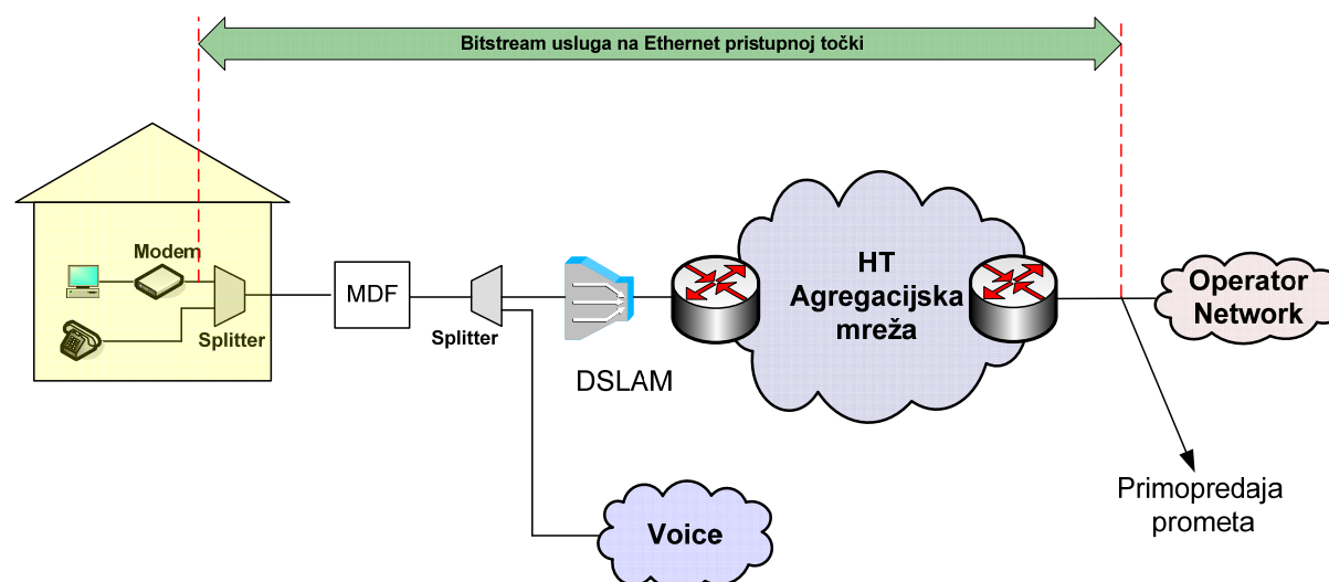
Slika 14. Veleprodajni širokopolasni pristup za pružanje VoIP usluge na Ethernet razini u slučaju kada krajnji korisnik ostvaruje Osnovni pristup mreži putem usluge HT-a
