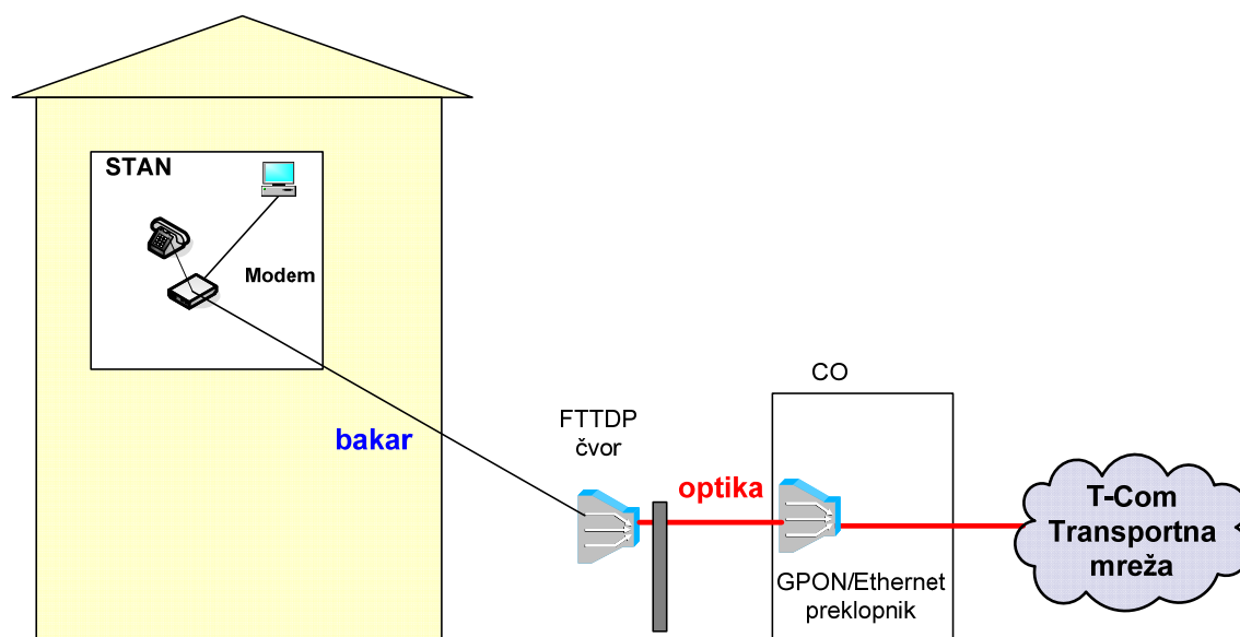
Slika 35. Način realizacije FTTP koncepta u pristupnoj mreži
