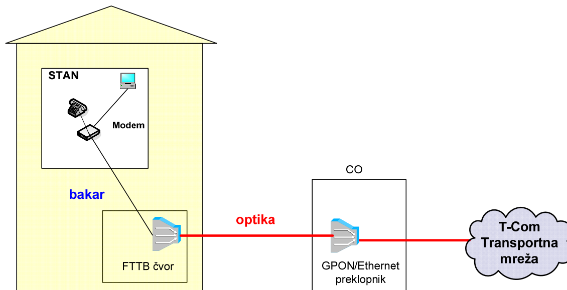
Slika 34. Način realizacije FTTB koncepta u pristupnoj mreži
