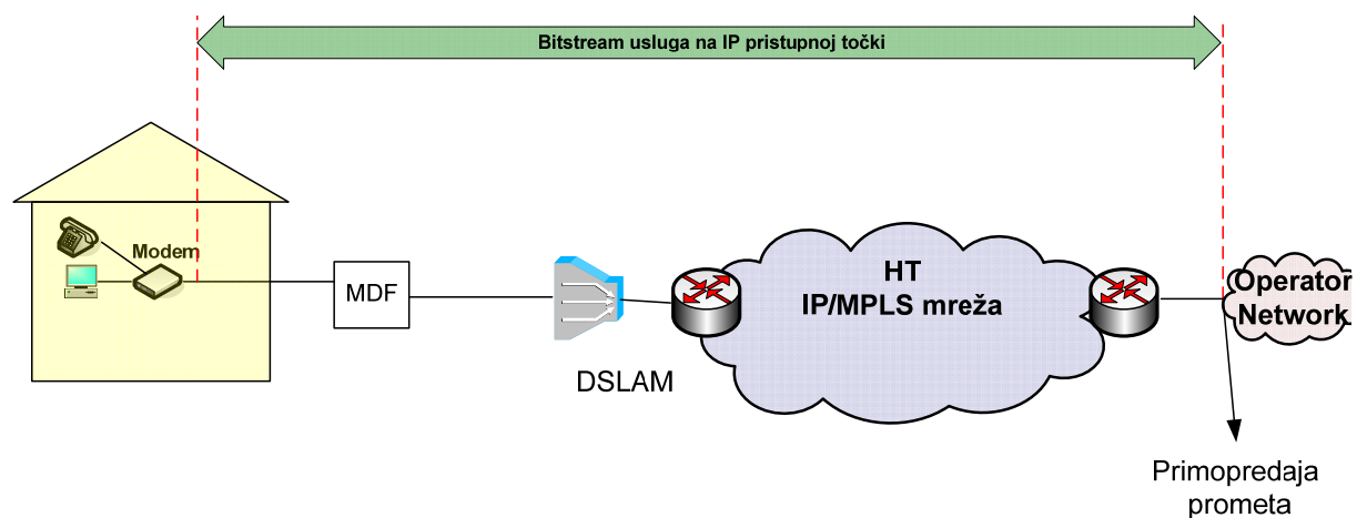
Slika 16. Veleprodajni širokopojsni pristup za pružanje VoIP usluge na IP razini u slučaju kada krajnji korisnik ostvaruje Osnovni pristup mreži putem usluge HT-a
