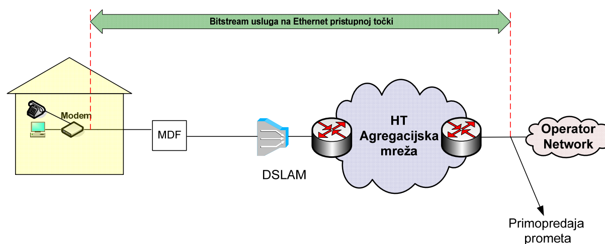
Slika 15. Veleprodajni širokopolasni pristup za pružanje VoIP usluge na Ethernet razini u slučaju kada krajnji korisnik ostvaruje Osnovni pristup mreži putem usluge Operatora korisnika
