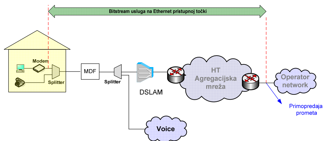
Slika 3. Veleprodajni širokopolasni pristup za pružanje Internet usluge na Ethernet razini u slučaju kada Krajnji korisnik ostvaruje Osnovni pristup mreži putem usluge HT-a.
