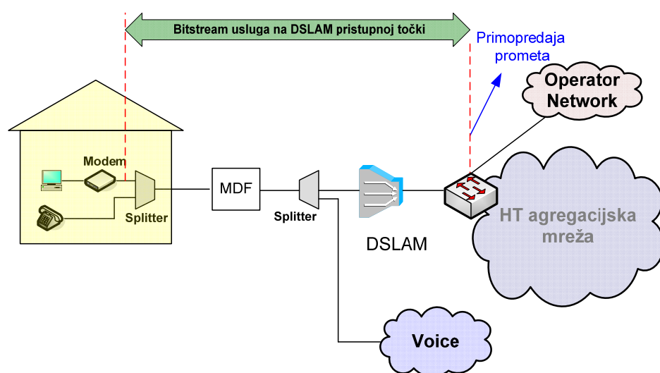
Slika 7. Veleprodajni širokopojasni pristup za pružanje Internet usluge na DSLAM razini u slučaju kada krajnji korisnik ostvaruje Osnovni pristup mreži putem usluge HT-a
